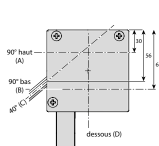
Sorties manivelle
