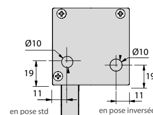
Sortie sur joue
