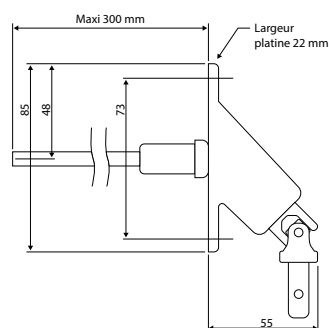
Sortie avec renvoi de manivelle
