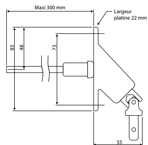
Sortie avec renvoi de manivelle
