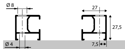
Pose de face vissée
