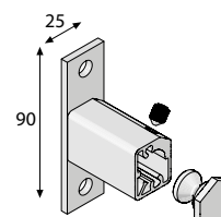
Pose face déportée
