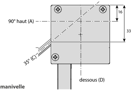
Sorties manivelle
