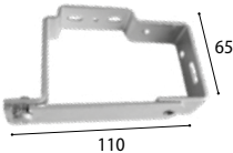
P2 Étrier de face
