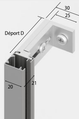
C2 Coulisses de face Avec équerres de déport (55 à 130 mm), coloris assorti aux lames.
