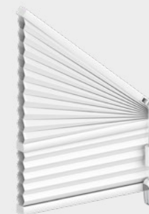
F3 Forme trapèze Avec frein. La manœuvre se situe toujours sur la petite hauteur. Guidage impossible. Lg maxi 1200 mm. Ht maxi 2300 mm. Prix store rectangle + prix store triangle + prix assemblage
