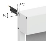
Sortie sur face arrière en pose standard
