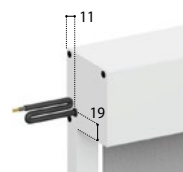
Sortie sur joue en pose standard
