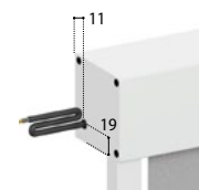
Sortie sur joue en pose inversée
