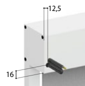
Sortie sur face arrière en pose inversée
