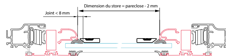
Prise de mesure avec ventouses
