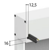
Sortie sur face arrière en pose inversée
