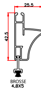
BARRE DE CHARGE
